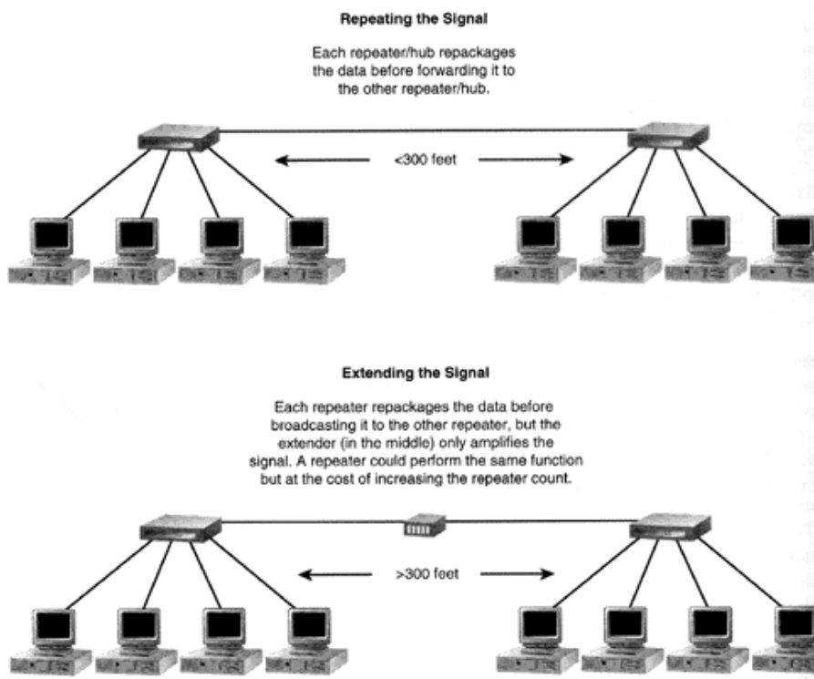
Figura 1 - Aplicação de repetidores
