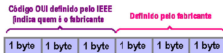
Figura 4 – Estrutura do endereço MAC segundo o IEEE
