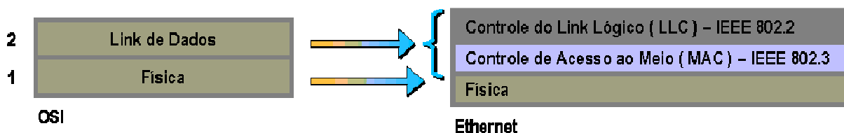
Figura 1 - Arquitetura Ethernet
