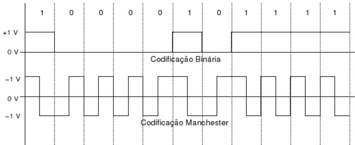
Figura 2 - Codificação Manchester
